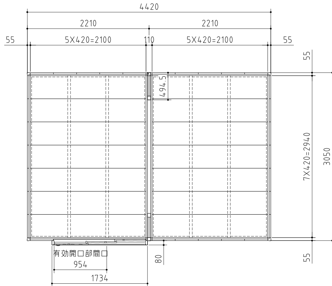
平面図
